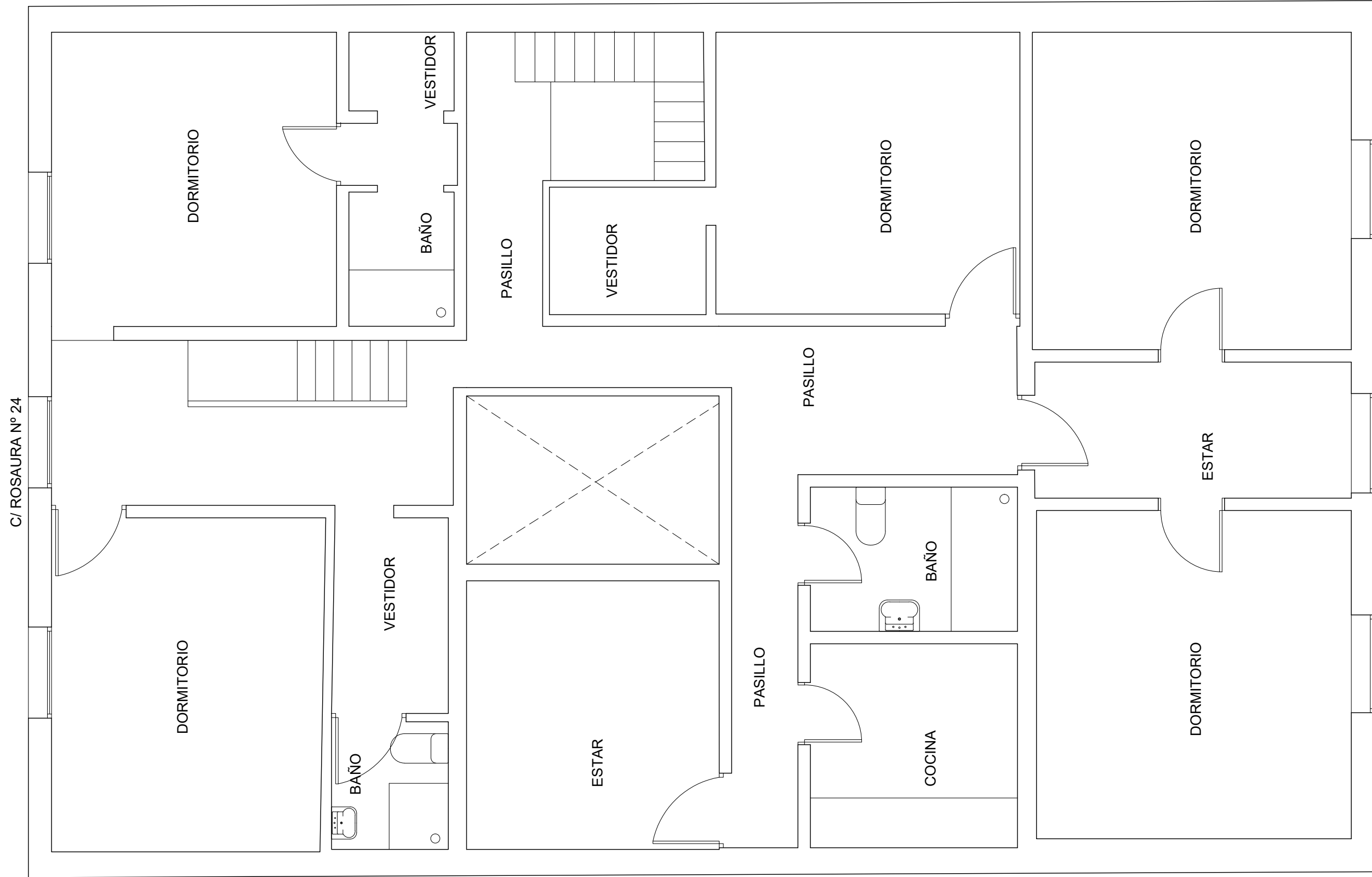
PLANTA ALTA
